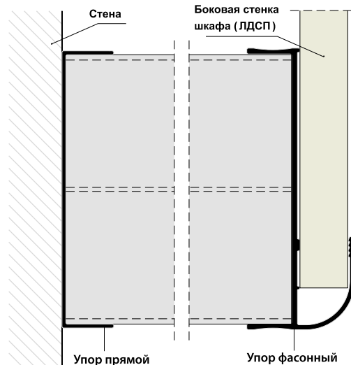
Вид сверху
